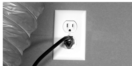
figure 9.2 Cordon électrique du VRC/VRE. Votre système est muni d'un fil de raccord pour une prise de 120 volts. Il est déconseillé d'utiliser un rallonge électrique pour connecter votre système. Si vous n'avez pas accès à une prise de courant avec un circuit distinct, il est recommandé de faire appel à un électricien pour en faire l'installation.
