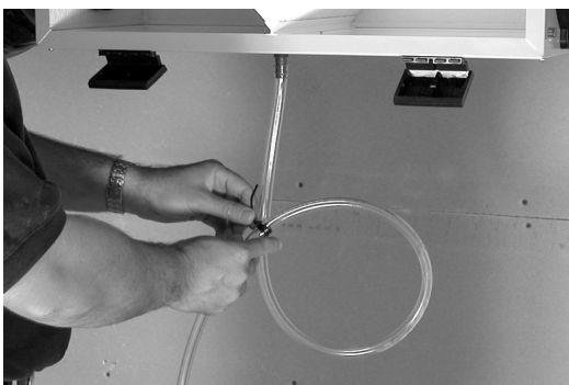
figure 8.1 Former un siphon dans le conduit.
