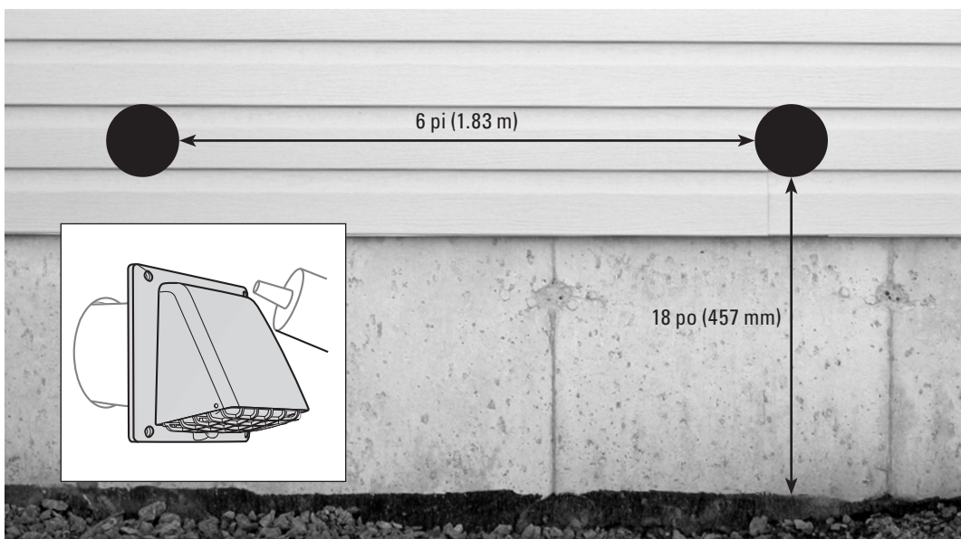
figure 10.1 Localiser l'emplacement des événements sur la maison.
