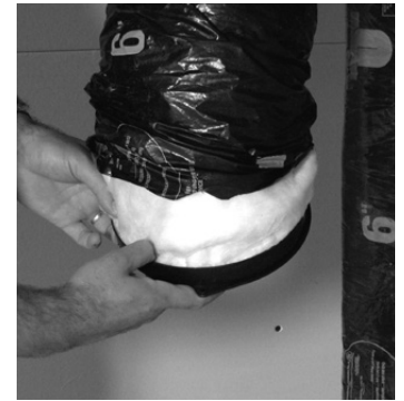
figure 7.2 Insérer la gaine isolante à l'intérieur de la double paroi du collet amovible.
